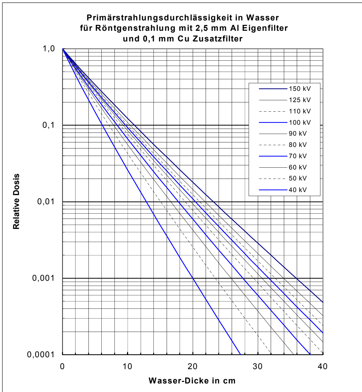
Abbildung A-3: Primärstrahlungstransmission in Wasser für Röntgenstrahlung mit Röhrensparnungen von 40 bis 150 kV und 2,5 mm Al Eigenfilter Eigenfilter und 0,1 mm Cu Zusatzfilter
