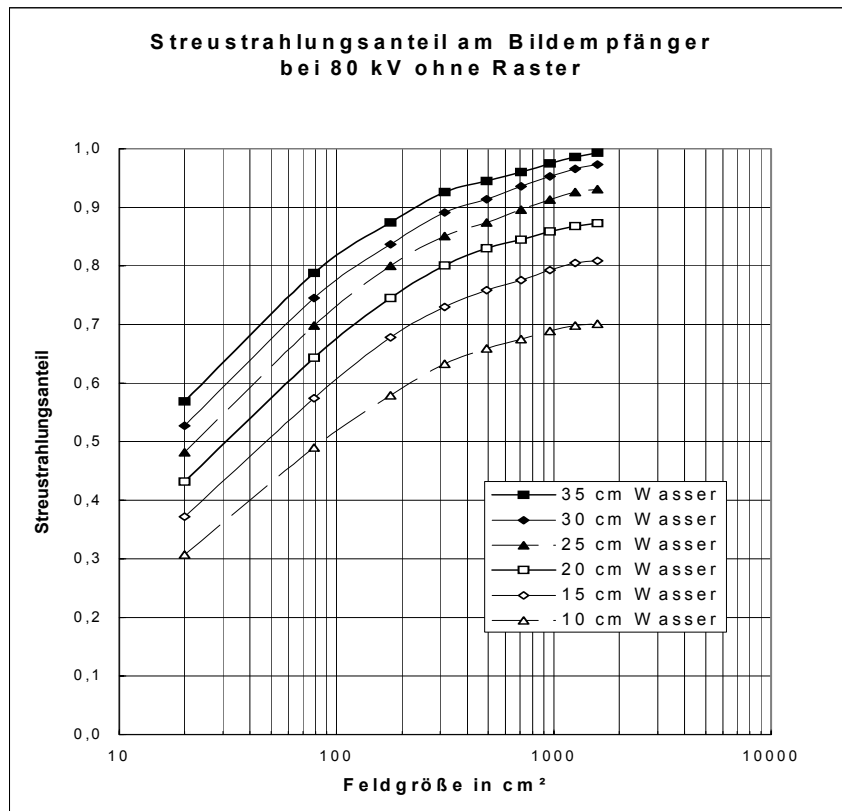
Abbildung A- 5: Streustrahlungsanteil der Nutzstrahlung am Bildempfänger bei 80 kV ohne Raster in Abhängigkeit von Feldgröße und Wasser-Phantomdicke
