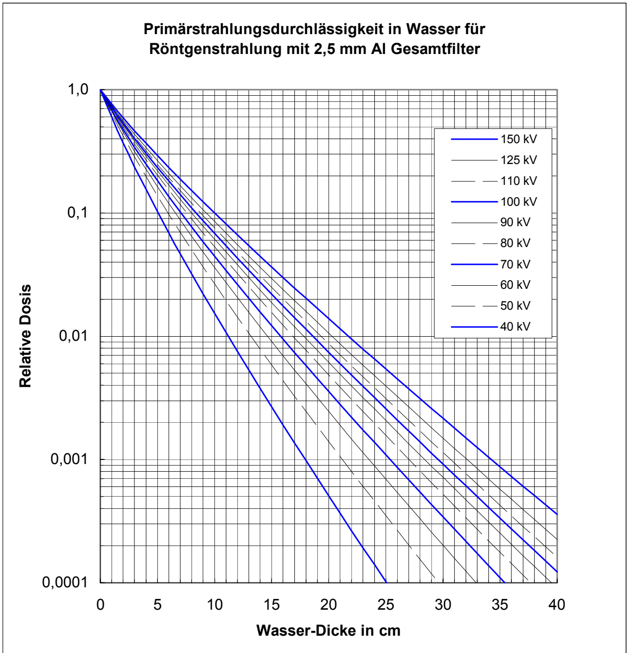
Abbildung A-2: Primärstrahlungstransmission in Wasser für Röntgenstrahlung mit Röhrenspannungen von 40 bis 150 kV und 2,5 mm Al Eigenfilter ohne Zusatzfilter
