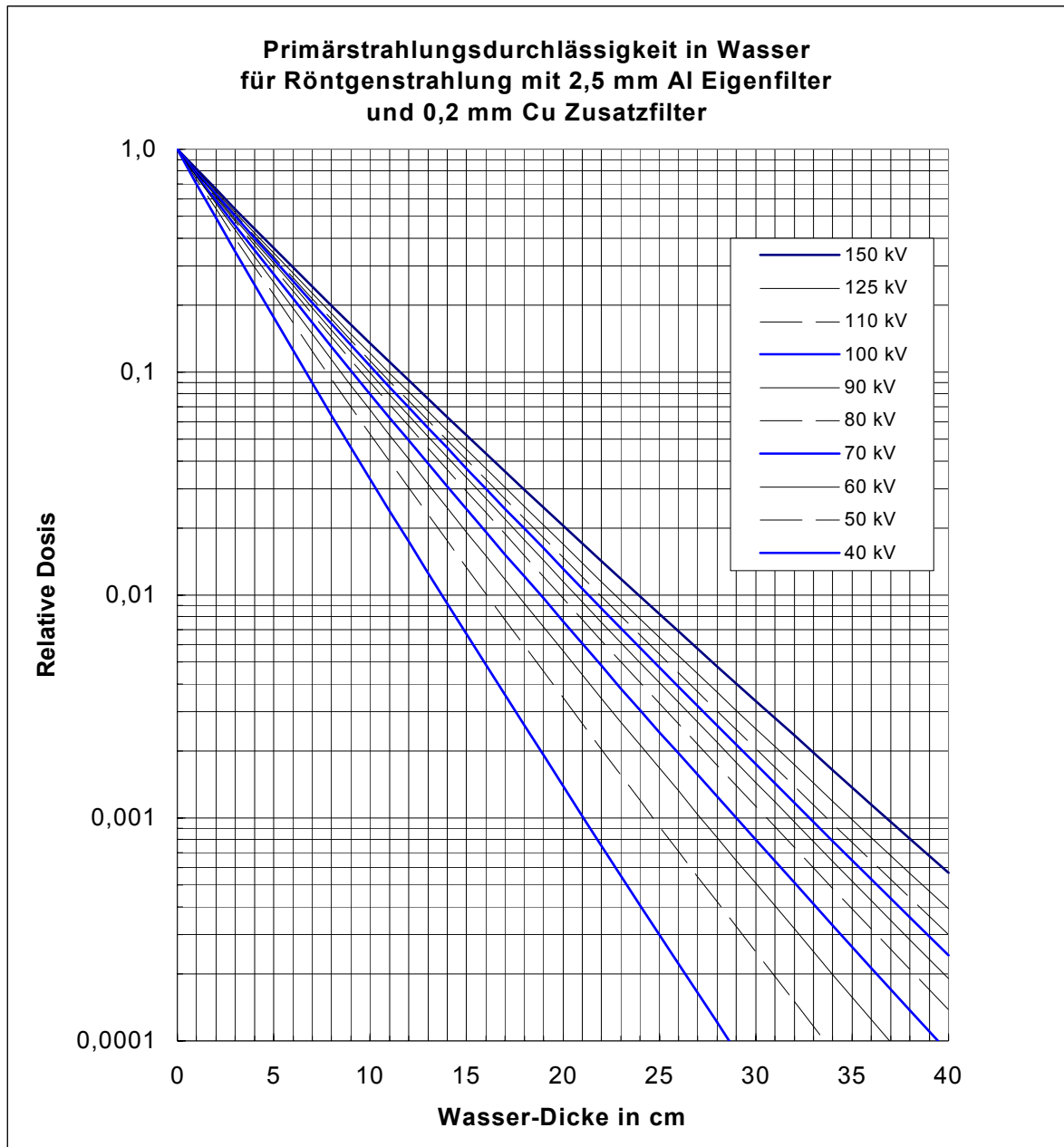
Abbildung A-3: Primärstrahlungstransmission in Wasser für Röntgenstrahlung mit Röhrensparnungen von 40 bis 150 kV und 2,5 mm Al Eigenfilter und 0,2 mm Cu Zusatzfilter
